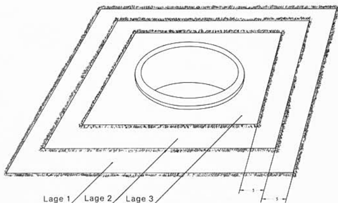
Laminatkragen. Alle Anschlüsse werden mit drei Lagen Glasmatte treppenförmig vorbeschichtet. Bei den Flächenbeschichtungen kann man dann später schneller arbeiten.
