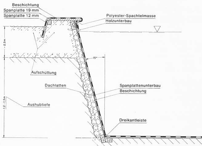
Spanplattenbecken im Schnitt
