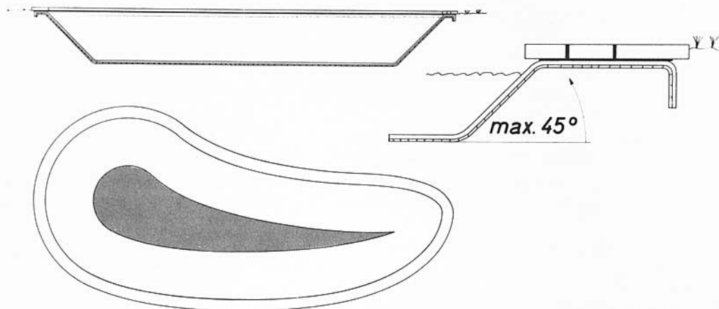
Zierteich mit Gips-Jute-Unterbau in Ansicht und Schnitt. Die Beckenwand ist unter 45^\circ geneigt, um den Erddruck auszuschalten. Mit diesem Unterbau können beliebig geformte Becken sehr preisgünstig hergestellt werden.
