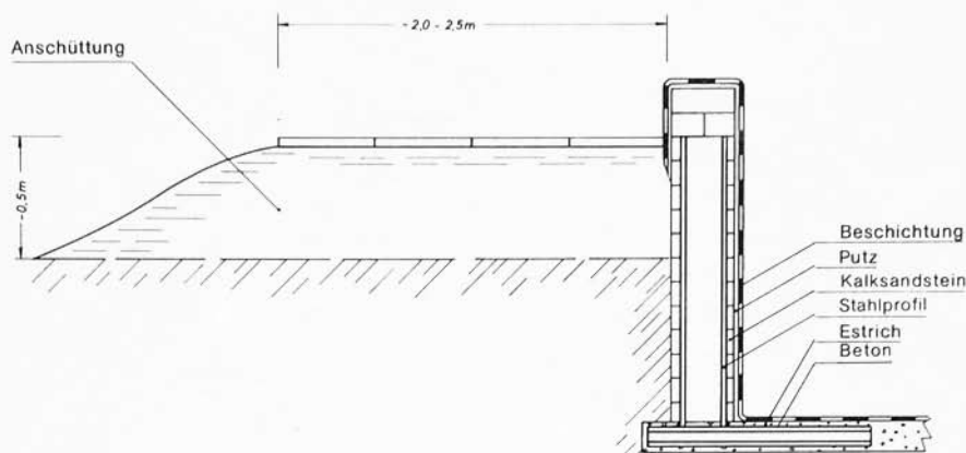
Ein Teil des Erdaushubs wird als Anschüttung verwendet. Im Wandschnitt ist der von uns lieferbare Stahlprofil-Winkel erkennbar.
