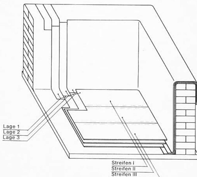
Bodenbeschichtung. Die Bahnen werden parallel zu den kurzen Beckenseiten verlegt. Im Boden werden drei Lagen naß-in-naß eingebracht.
