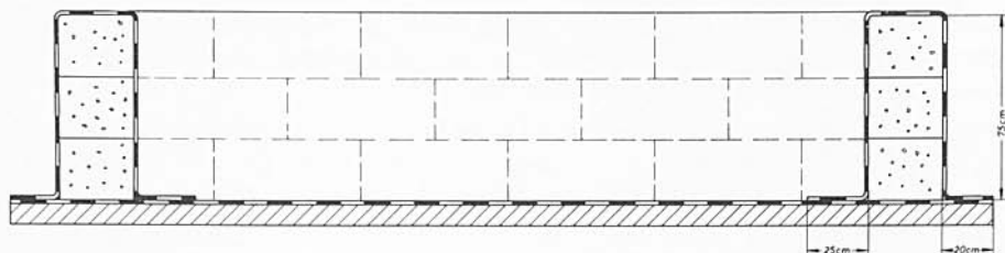
Flachwasserbecken mit 65 cm Füllhöhe. Die Leichtbausteine sind mit FLEXOVOSS K 6 TT einfach verklebt und anschließend mit 3 Lagen Glasmatte und Polyesterharz übertapeziert worden.
